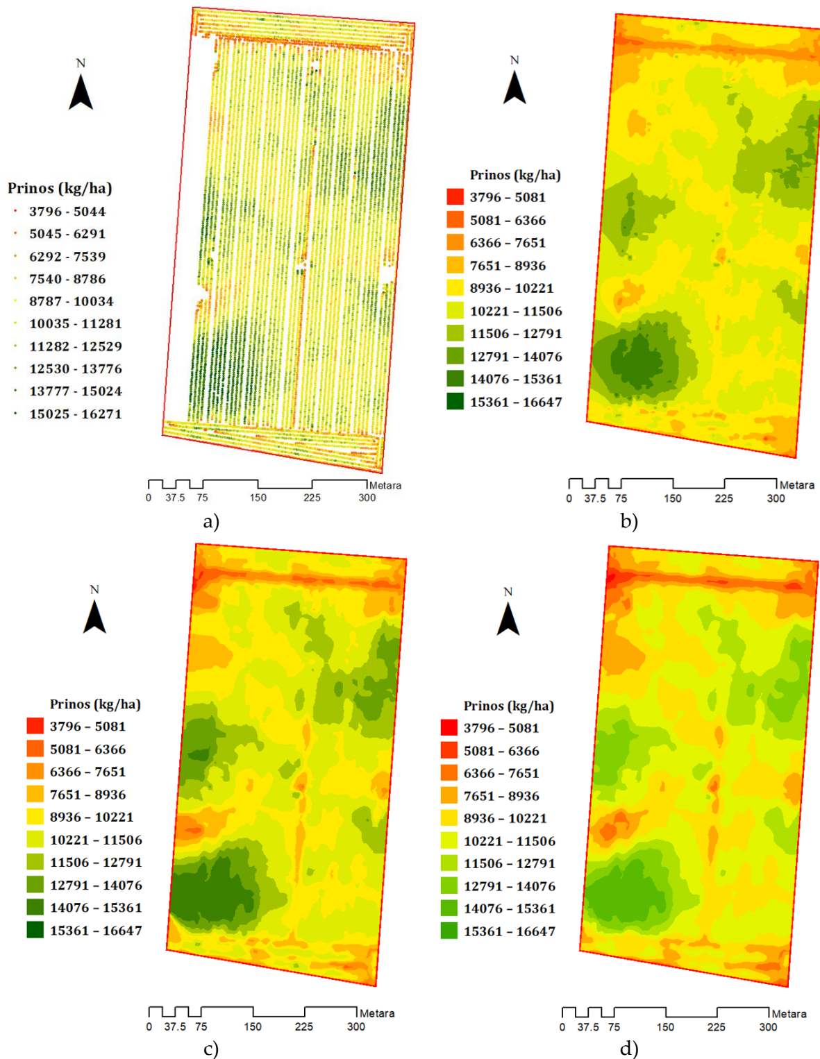
Slika 1.5. Mape prinosa kukuruza izrađene različitim metodama prostorne interpolacije: a) Podaci sa monitora prinosa; b) Usrednjavanje; c) Ponderisanje recipročno rastojanju; d) Kriging (zapis sa kombajna firme Agropromet d.o.o., Bečej)
